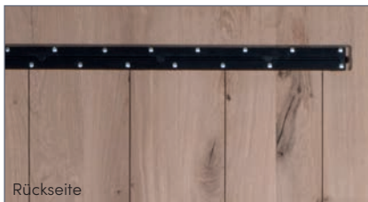
Rückseite Stahlprofile & Entlastungsgrillen
